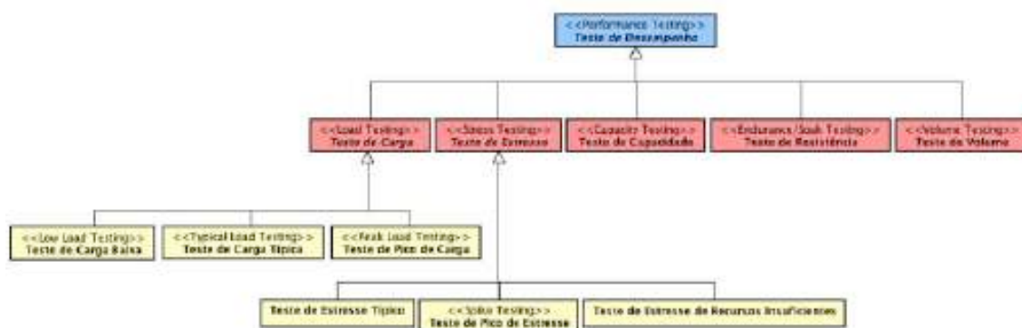
Figura 5.4: Tipos de testes de desempenho.
